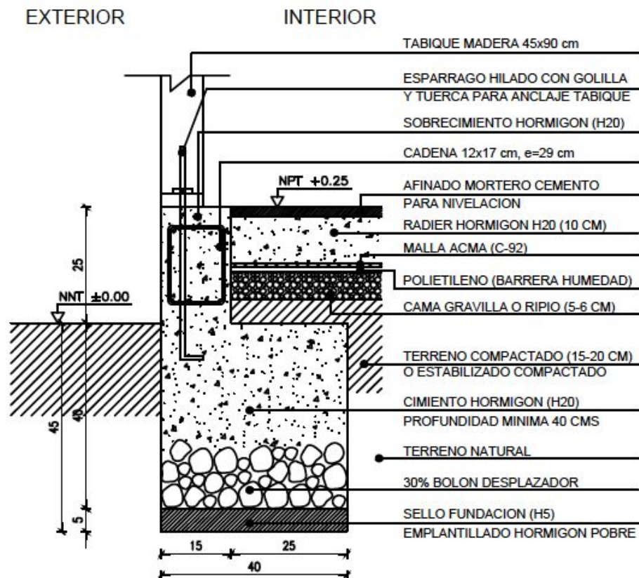
DET. 1 FUND. TIPO
